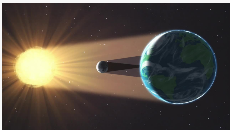
Diagrama de la Tierra, la Luna y el Sol durante el eclipse total
