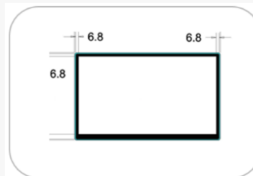
6.8mm Narrow bezel
