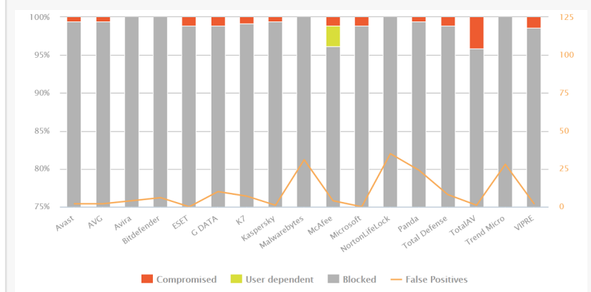
AV-Comparatives Test-Ergebnisse Q1 2022 - Real-World Protection Test von 17 Anti-Virus Produkten für Endverbraucher
