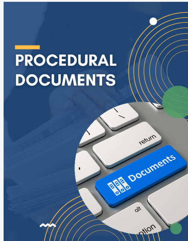
Spectrum EEO
