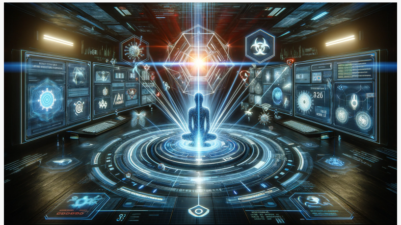
AI Protection
