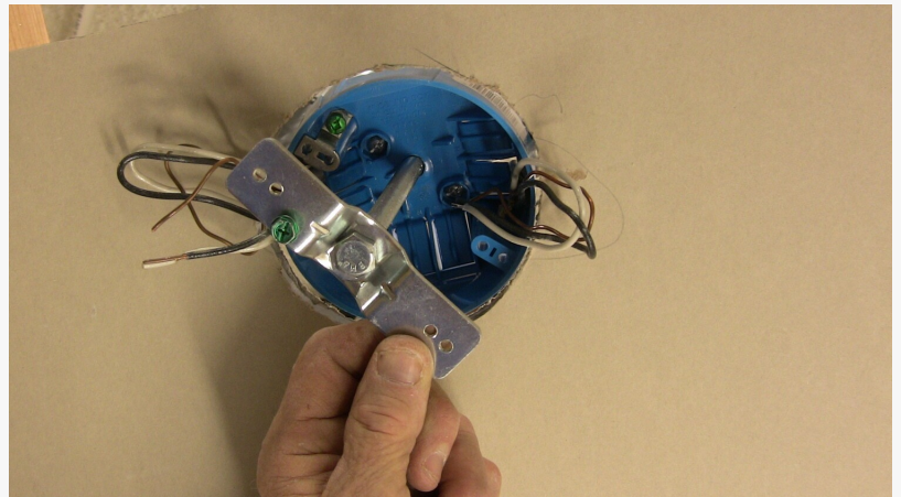
Ez brace bracket
