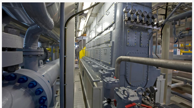
Laby compressor in LNG terminal
