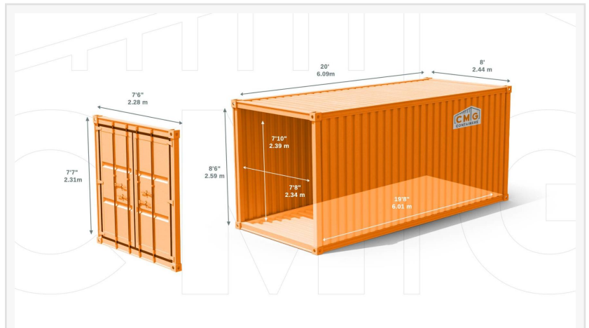
20ft-CMG-Container-for-sale
